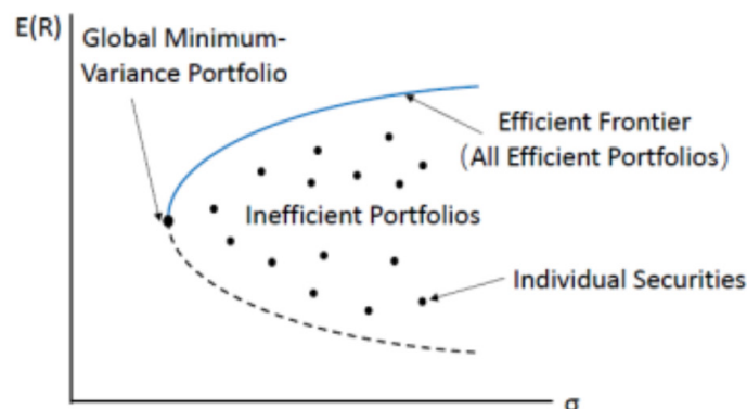
Fig. 1 Efficient Frontier [13].
